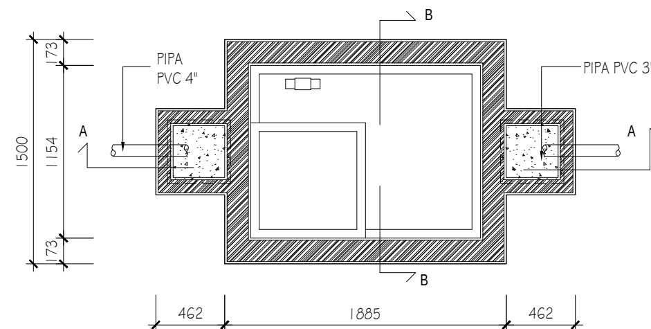
TAMPAK ATAS 1:50
